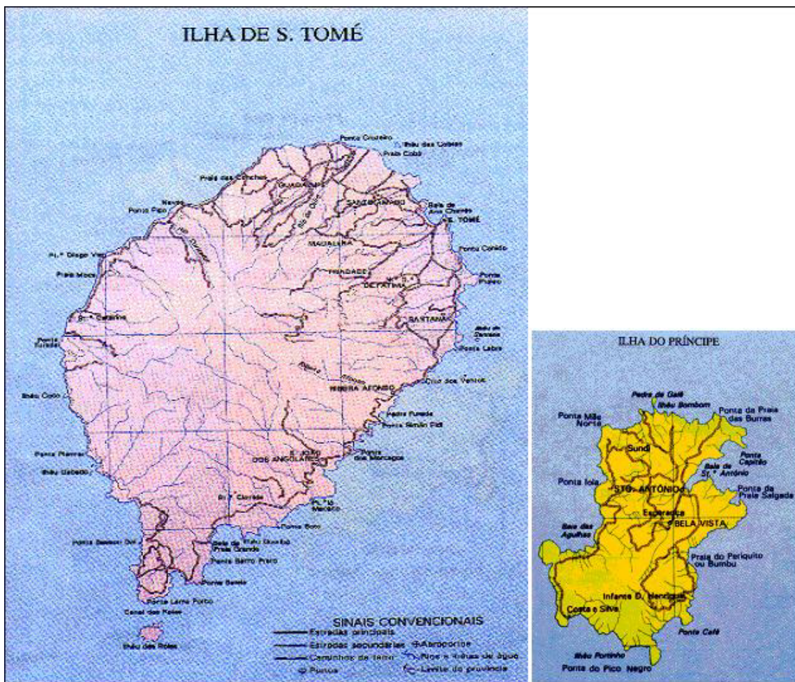
Figure 56: Carte Hydrographique de São Tomé et Príncipe
