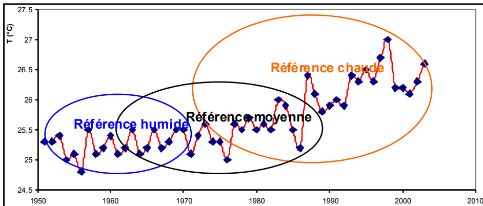
Figure 10 : Analogie thermique de 1951 à 2003 (à Sao Tomé, station de l'aéroport)
