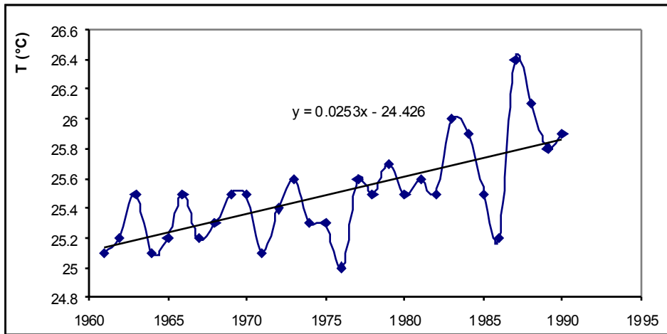
Figure 14: Tendence évolutive des températures (analogue sèche)
