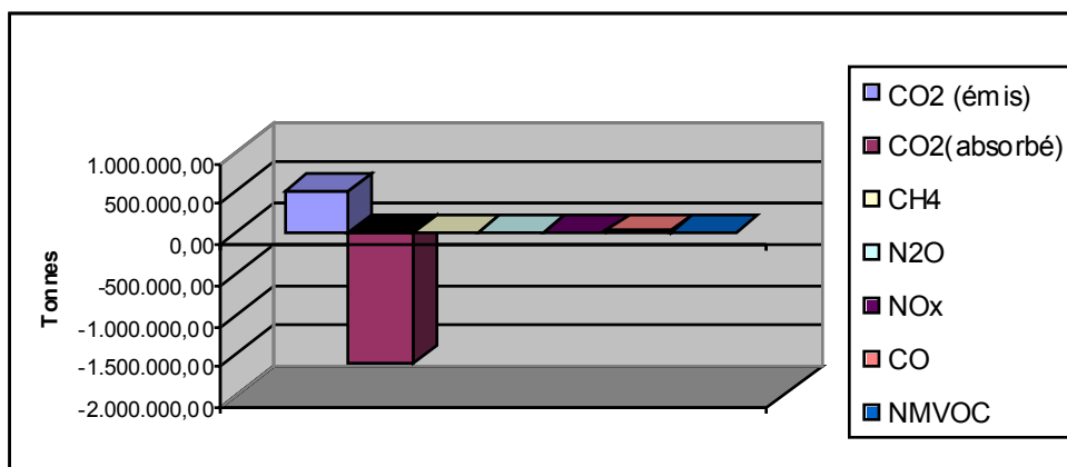
Figure 6 : Synthèse des émissions de GES
