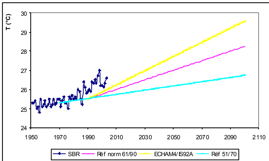
Figure 20 : Modifications probables des températures à l'horizon 2100
