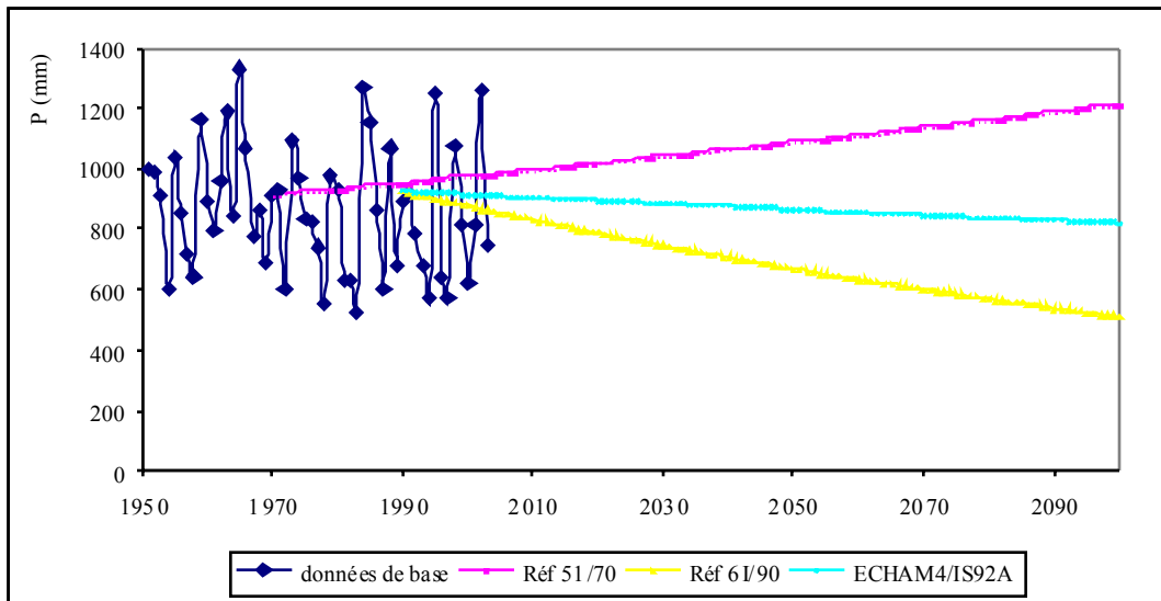
Figure 21 : Modifications probables des précipitations à l'horizon 2100
