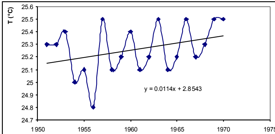
Figure 12 : Tendance évolutive des températures (analogie humide)
