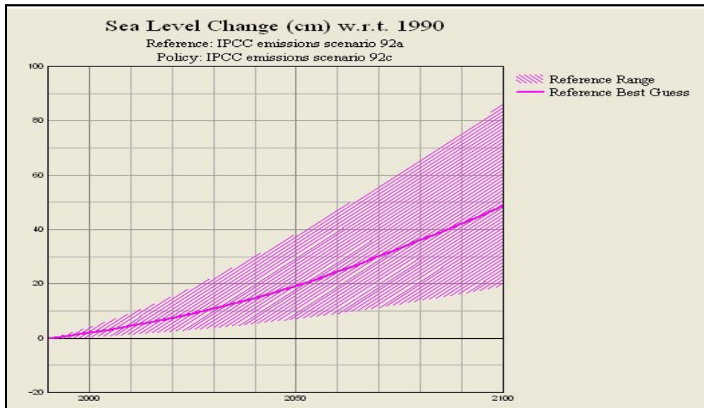
Figure 22 : Scénario d'évolution du niveau marin à l'horizon 2100
