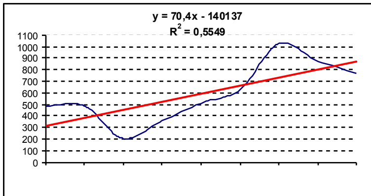
Figure 25 : évolution des coupes du bois dans les forêts d'ombrage
