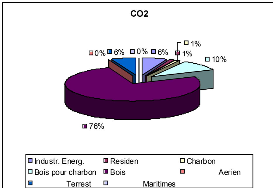
Figure 2 : Emissions du CO 2 du secteur énergie
