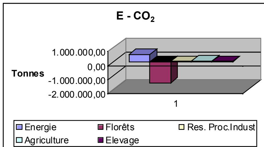
Figure 1: Bilan des émissions et des absorptions de carbone en E-CO 2
