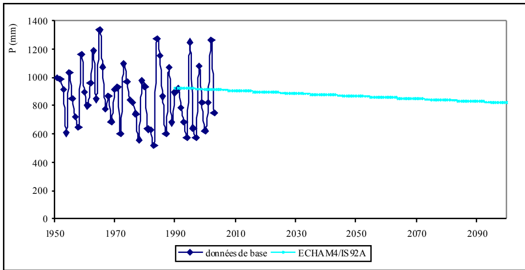
Figure 18 : Génération du changement des précipitations à l'horizon 2100 par le scénario de changement climatique IS92A. Avec modèle climatique ECHAM4
