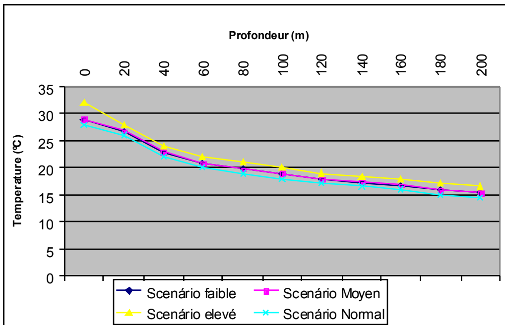
Figure 36 : Scénario de variation de la température à la surface pour l'année 2050
