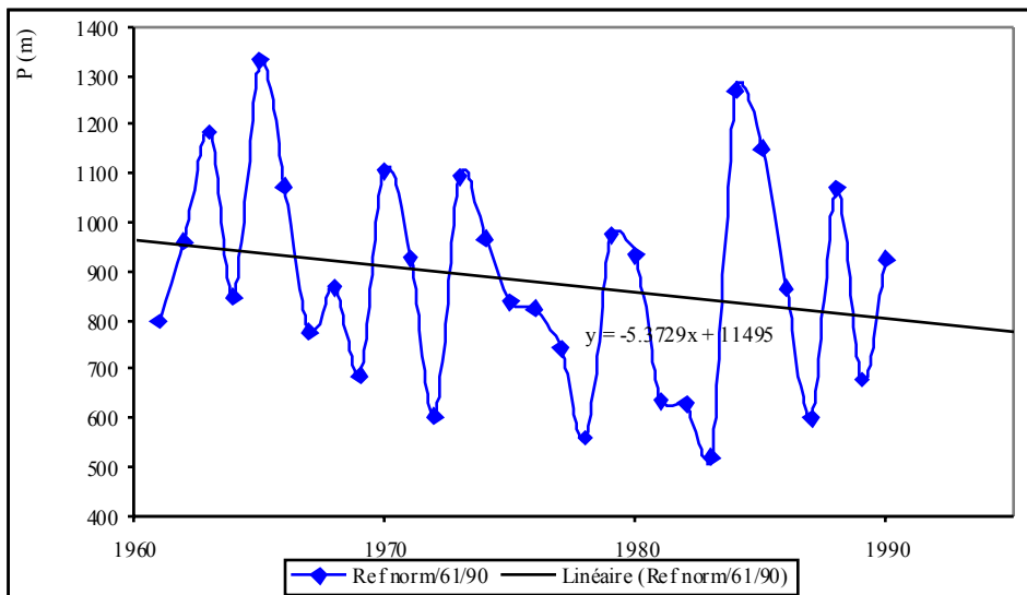
Figure 15: Tendence évolutive des précipitations (analogue sèche)
