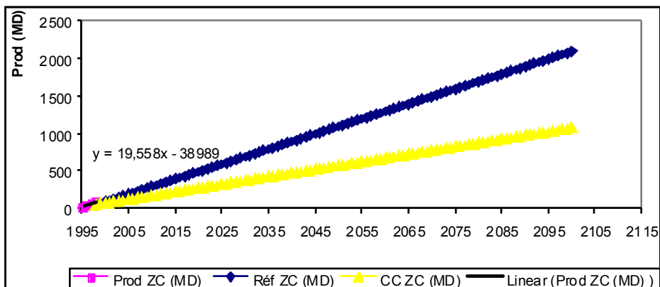
Figure 38 : Impact économique du changement climatique sur les ressources côtières à l'horizon 2100
