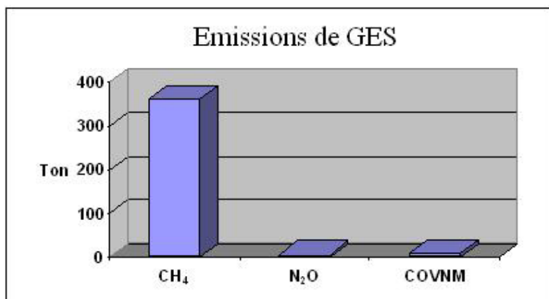
Figure 5 : Émissions du secteur de Résidus et Procédés Industriels
