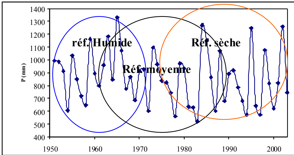
Figure 9 : Analogies pluviométriques de 1951 à 2003 (à Sao Tomé, station de l'aéroport)
