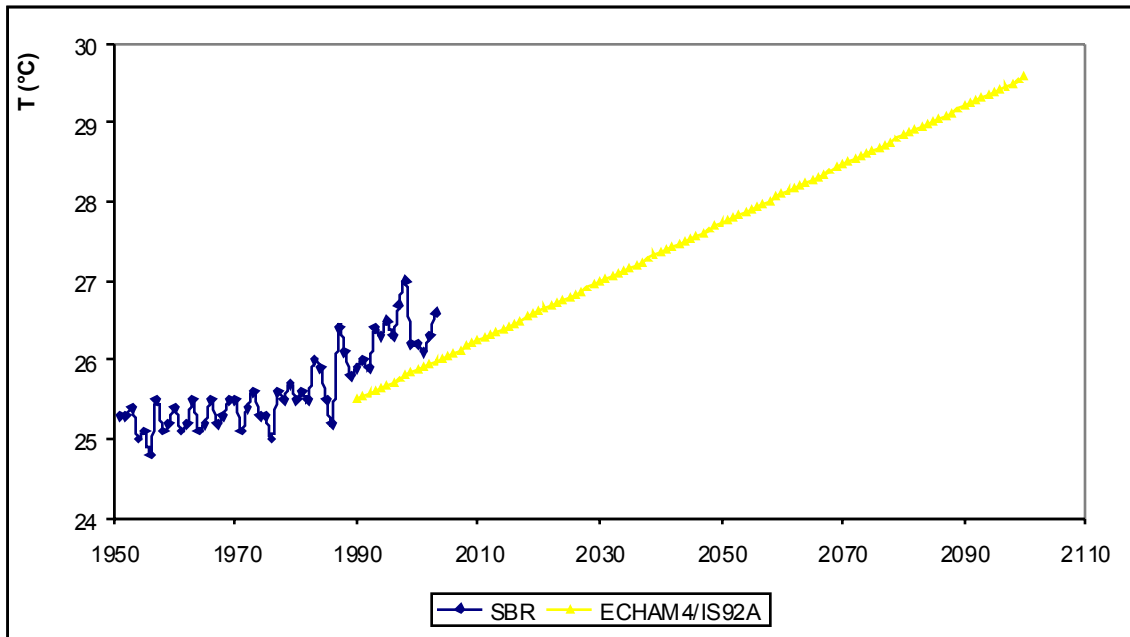
Figure 19 : Génération du changement des températures à l'horizon 2100 par le scénario de changement climatique IS92A. Avec modèle climatique ECHAM4
