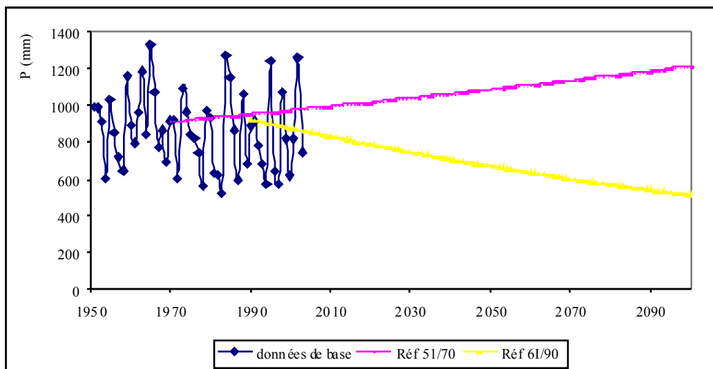
Figure 16 : Référence de base future des précipitations (pour un scénario humide et un scénario sec) à l'horizon 2100
