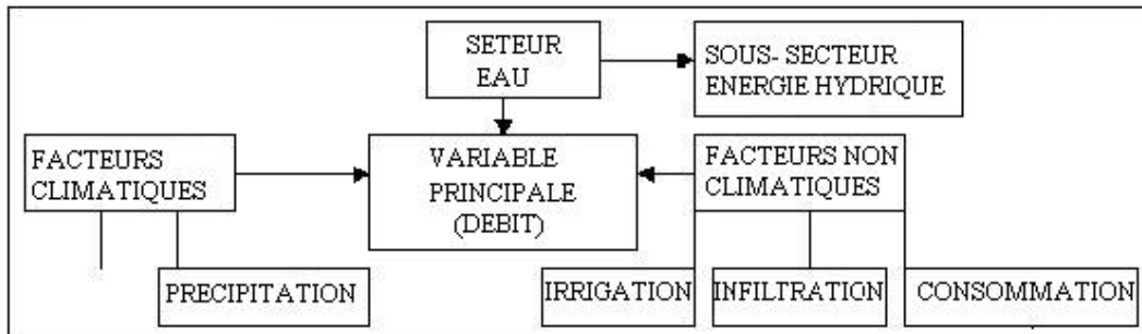
Figure 57 : Organigramme des influences des facteurs climatiques et non climatiques sur les ressources hydro-énergétiques.
