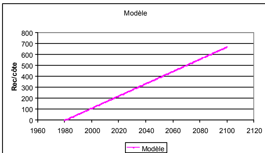
Figure 32 : Scénario avec changements climatiques pour la Zone Côtière
