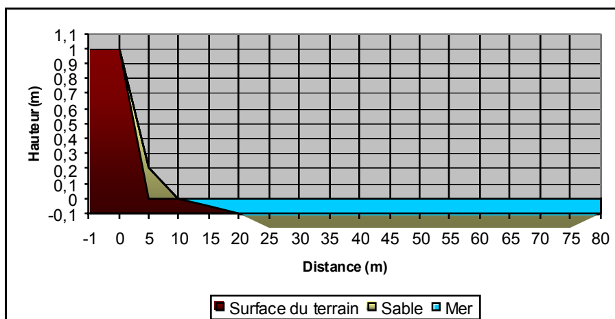
Figure 28–Schéma de la ligne de côte de la plage Diogo Nunes (S. Tomé), nouvelle position en 2003 indiquant une pénétration de plus de 100 m en 23 ans
