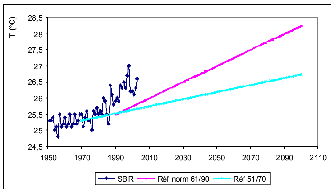
Figure 17 : Référence de base future des températures (pour un scénario humide et un scénario sec) à l'horizon 2100
