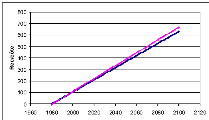
Figure 34 : Impact du changement climatique sur la dynamique du trait de côte à l'horizon 2100
