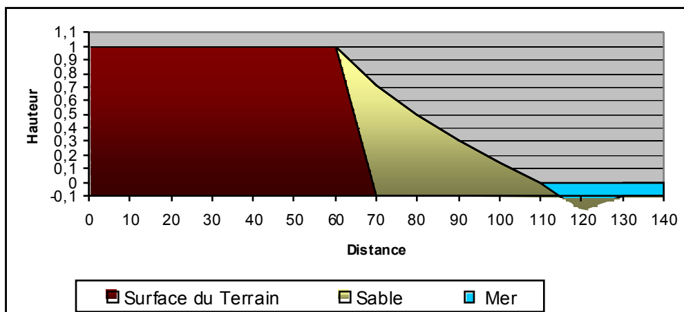
Figure 27 : Schéma de la ligne de côte de la plage Diogo Nunes (S. Tomé), position initiale du littoral en 1980 situé à 115 m du repère 0m
