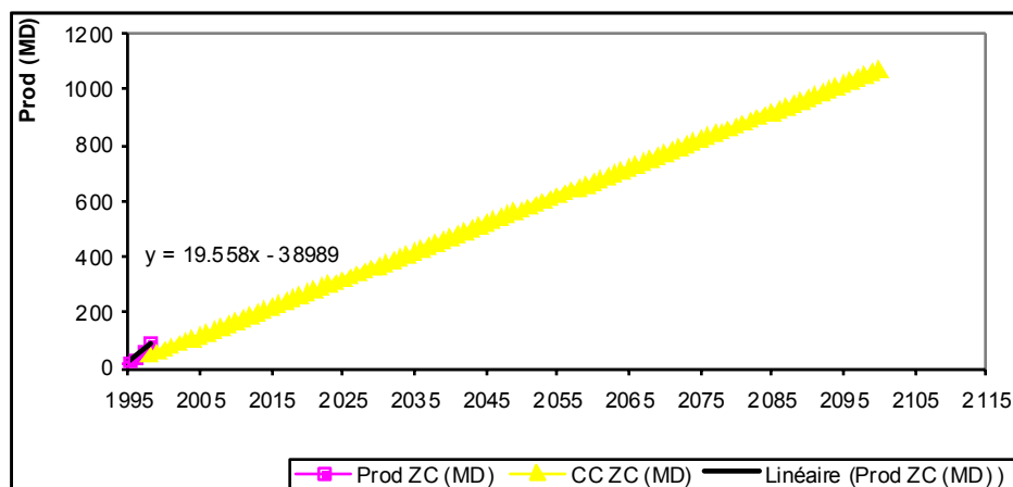
Figure 33 : Niveau des productions côtières en cas de changement climatique
