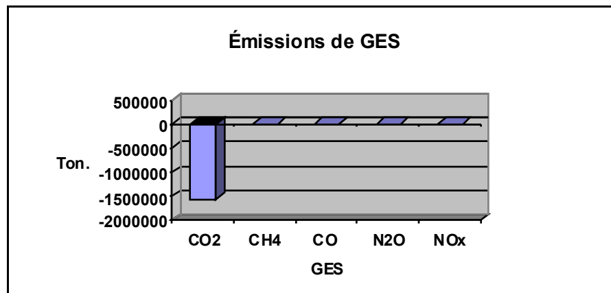
Figure 4: Synthèse des émissions du secteur des forêts
