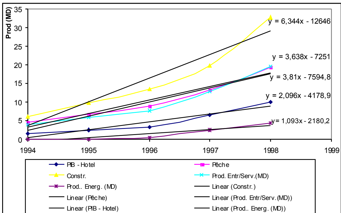
Figure 29: Situation de base actuelle et tendances évolutive des principaux secteurs économiques de la zone côtière
