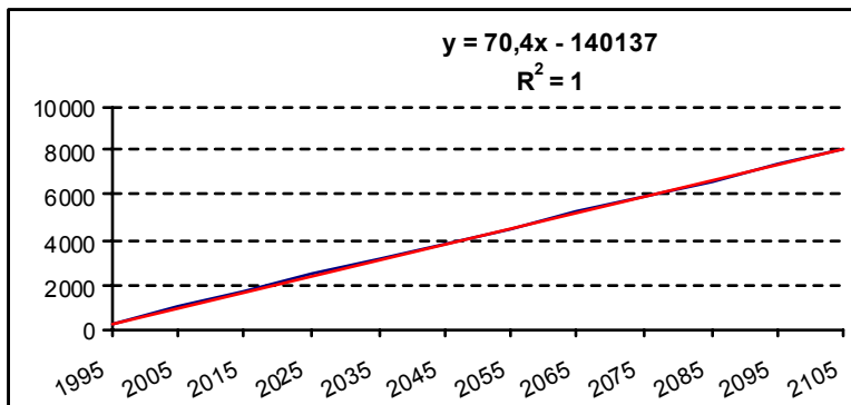
Figure 26 : référence de base future de l'exploitation du bois de qualité
