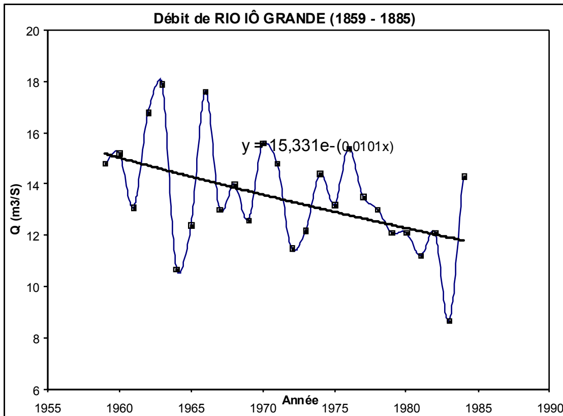
Figure 58 : Situation des écoulements de la rivière Iô Grande
