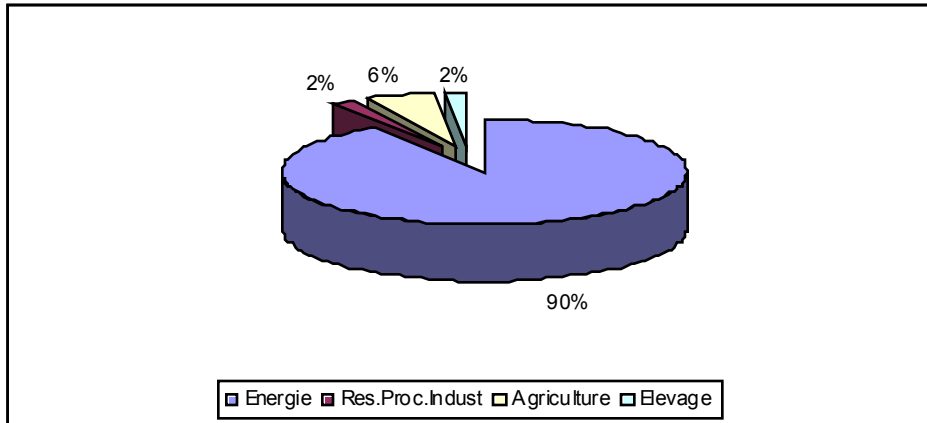
Figure 8 : Synthèse des émissions en E-CO 2
