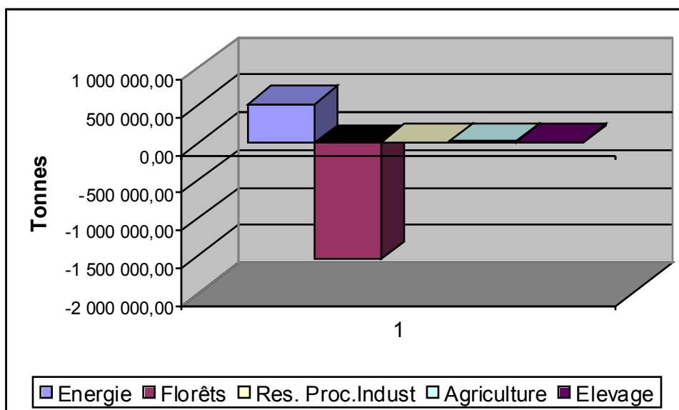
Figure 7 : Bilan des émissions de GES en E - CO 2
