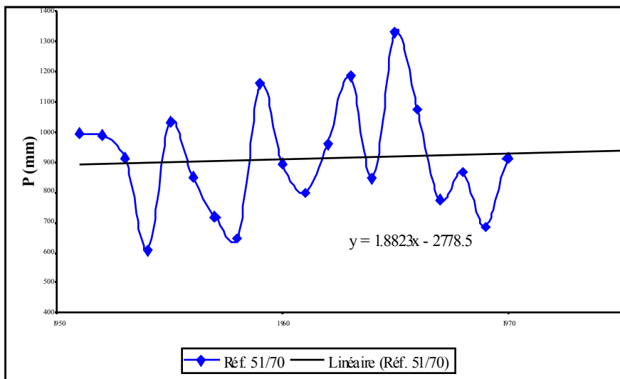
Figure 13: Tendance évolutive des précipitations (analogie humide).
