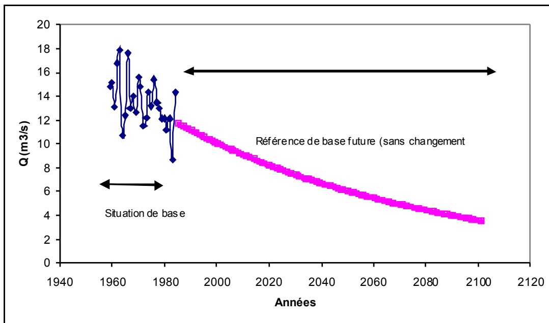
Figure 59: Référence future de l'évolution des écoulements
