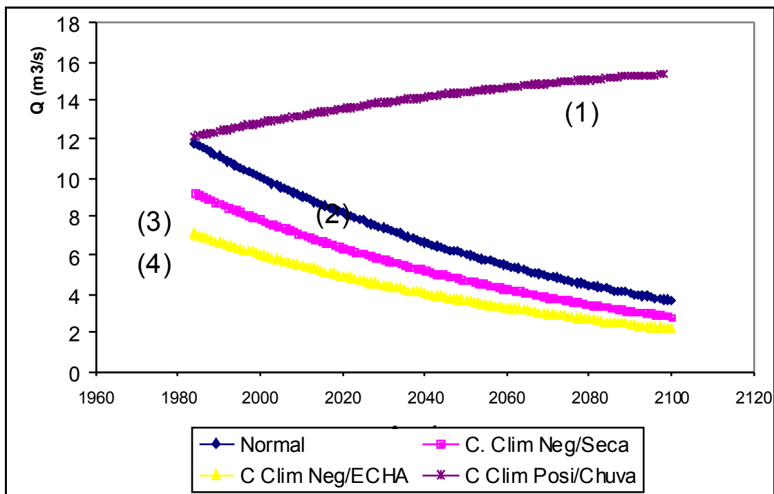
Figure 60 : Evolution comparée des références futures avec le scénario de changement climatique
