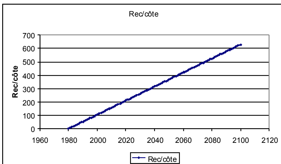
Figure 30 : Pénétration du trait de côte à l'horizon 2100 du fait de l'extraction des inerts côtiers
