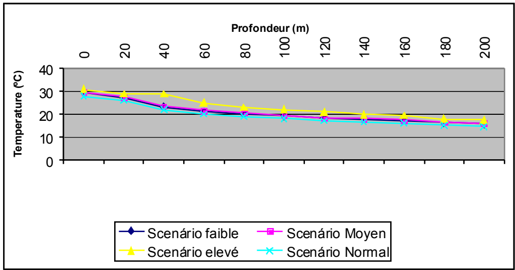
Figure 37 : Scénario de variation de la température des eaux marines à l'année 2100
