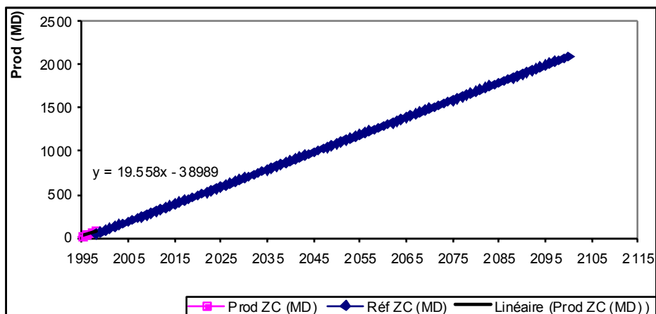
Figure 31 : Référence de base future des productions de la zone côtière à l'horizon 2100
