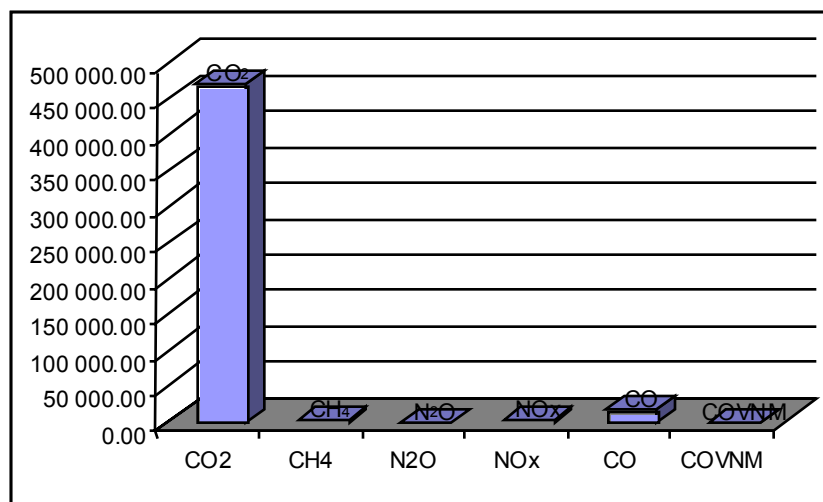
Figure 3 : Emissions de GES dans le secteur énergie
